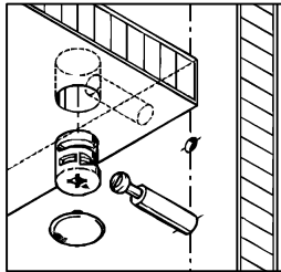
Вид Е
