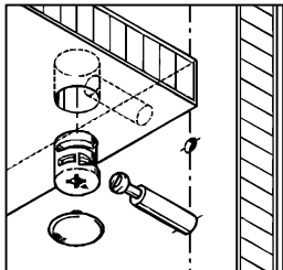
Вид Д
