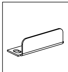
Вид И
