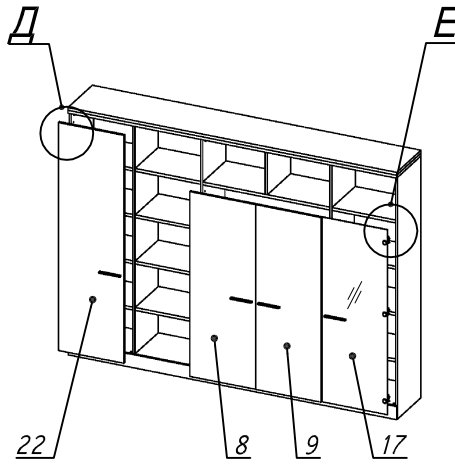
Вид Б
