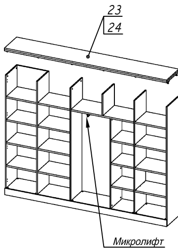
Вид А
