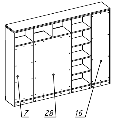
Вид Д
