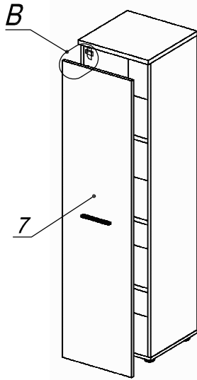
Вид Г
