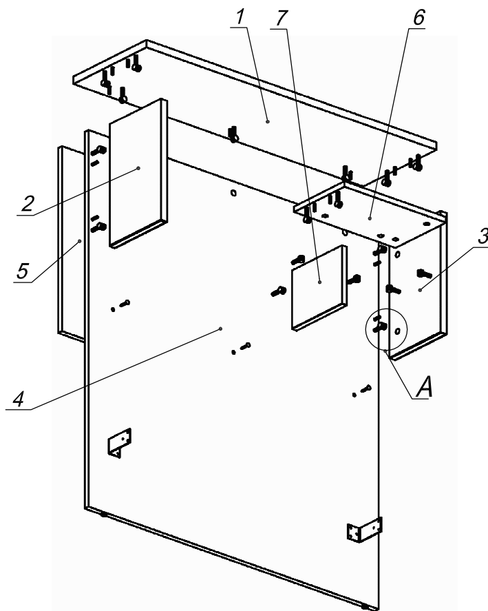
Схема сборки
