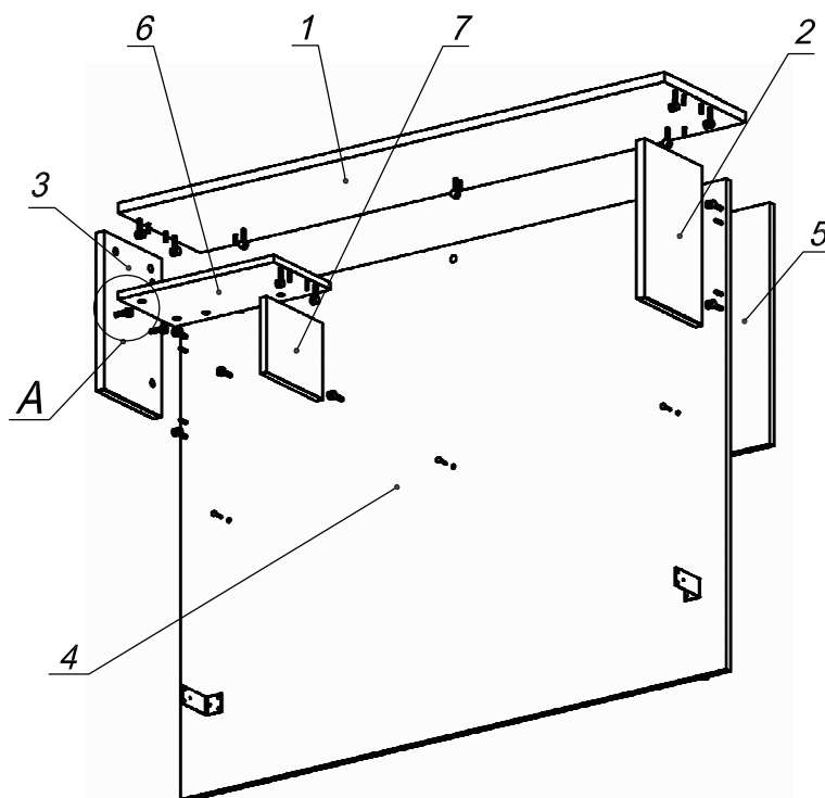
Схема сборки
