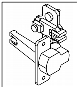
Вид В
